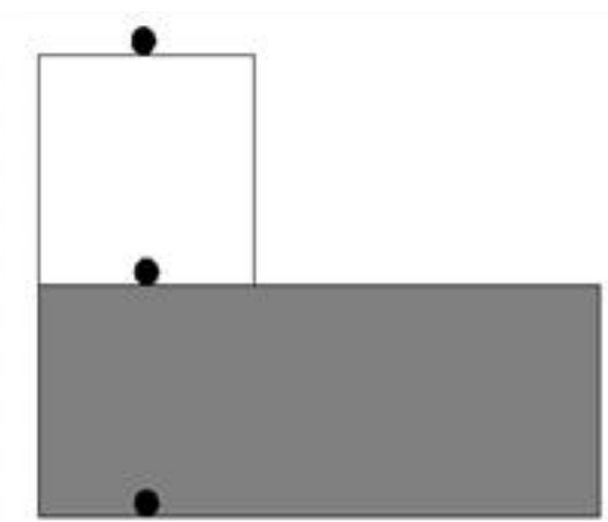
[별도 4] 중량이 급격하게 변하는 건축물의 지진가속도감지기 설치 위치(제15조 관련)
